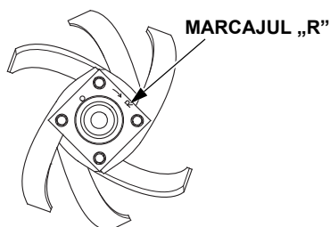
FREZĂ INTERIOARĂ, DREAPTA (vedere din partea dreaptă)
