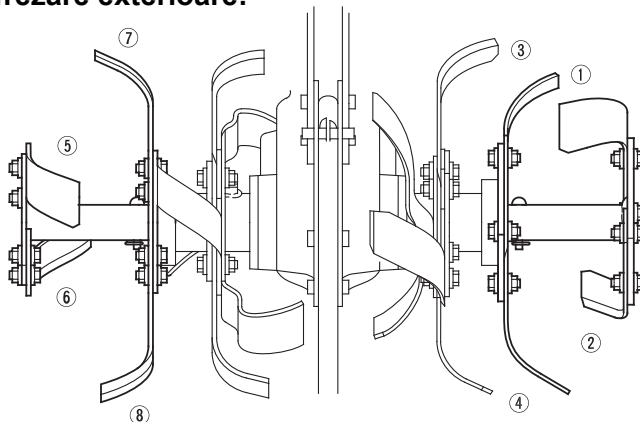
FREZĂ EXTERIOARĂ, DREAPTĂ (vedere din partea dreaptă)
