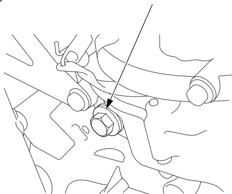
ȘURUB DE VERIFICARE A NIVELULUI DE ULEI DE AMBREIAJ
