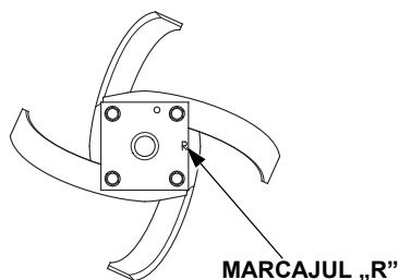
FREZĂ EXTERIOARĂ, DREAPTA (vedere din partea dreaptă)
