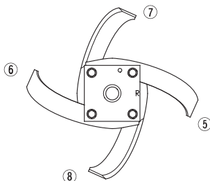
FREZĂ EXTERIOARĂ, DREAPTĂ (vedere din partea dreaptă)
