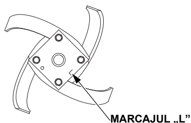
FREZĂ EXTERIOARĂ, STÂNGA (vedere din partea stângă)
